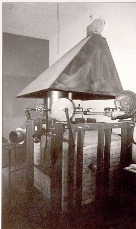
Labe honek hondarra beira bihurtzea lortzen du, 1.400 gradutan.
