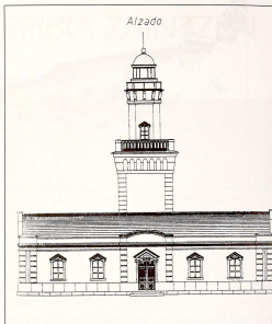
Autocad programaren bidez egina, Lafarga-ren proiektutik abiatuta. Eglea: J.L. Noain
